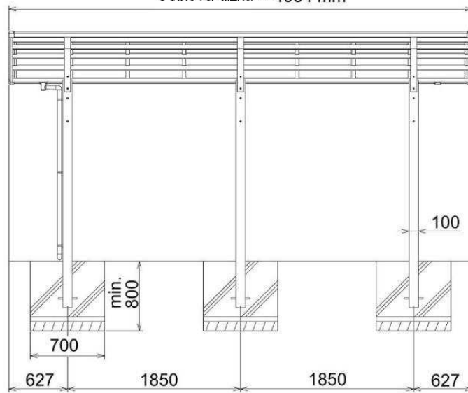
↑ Pohľad B
